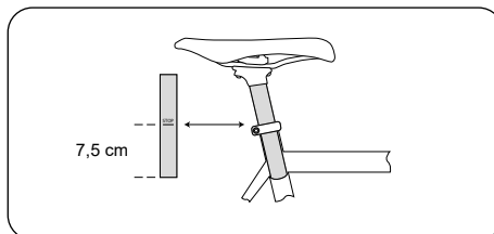
Höhenverstellung möglich
