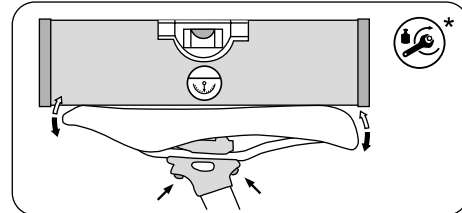
Patentstütze mit Zweischaubefestigung
